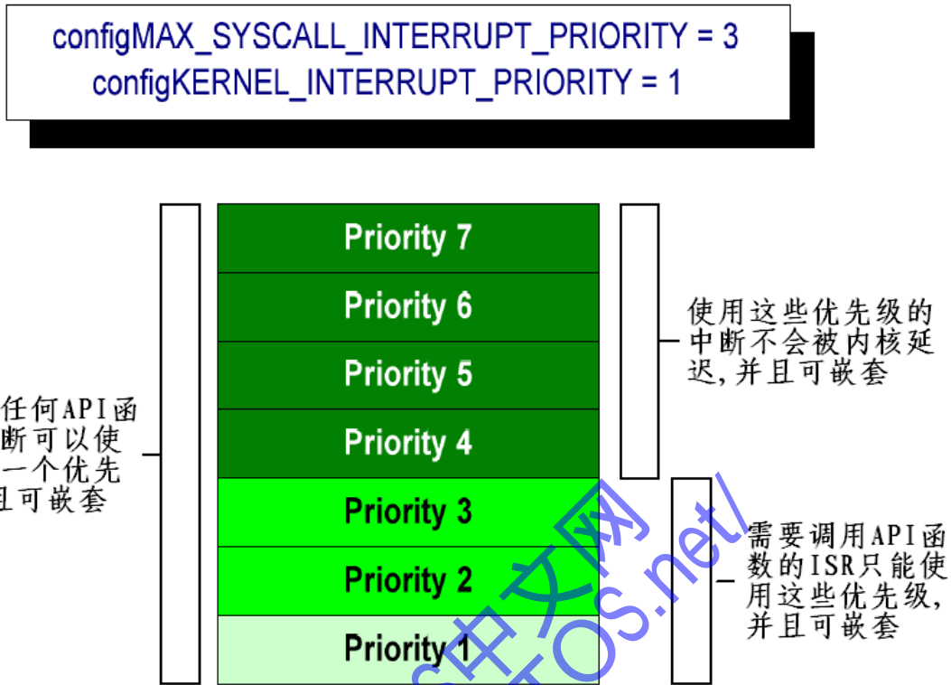
图 35 中断控制常量影响中断嵌套行为
